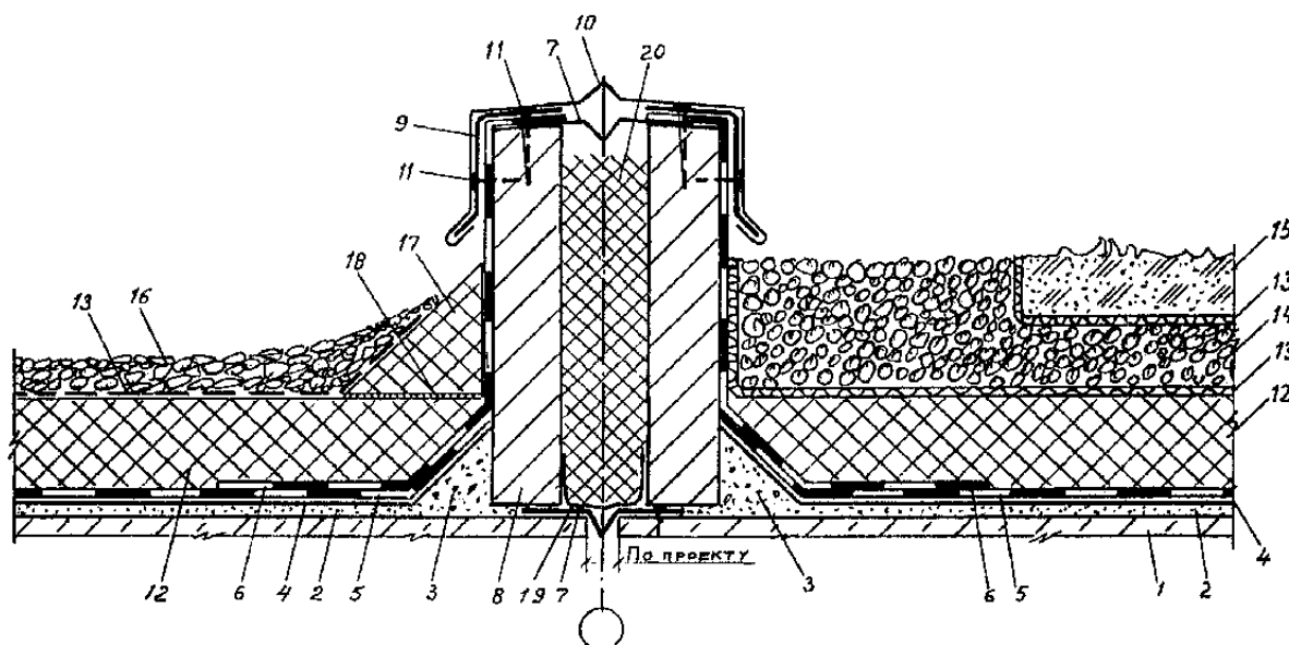
Рис. 6 Деформационный шов при инверсионной эксплуатируемой кровле.
