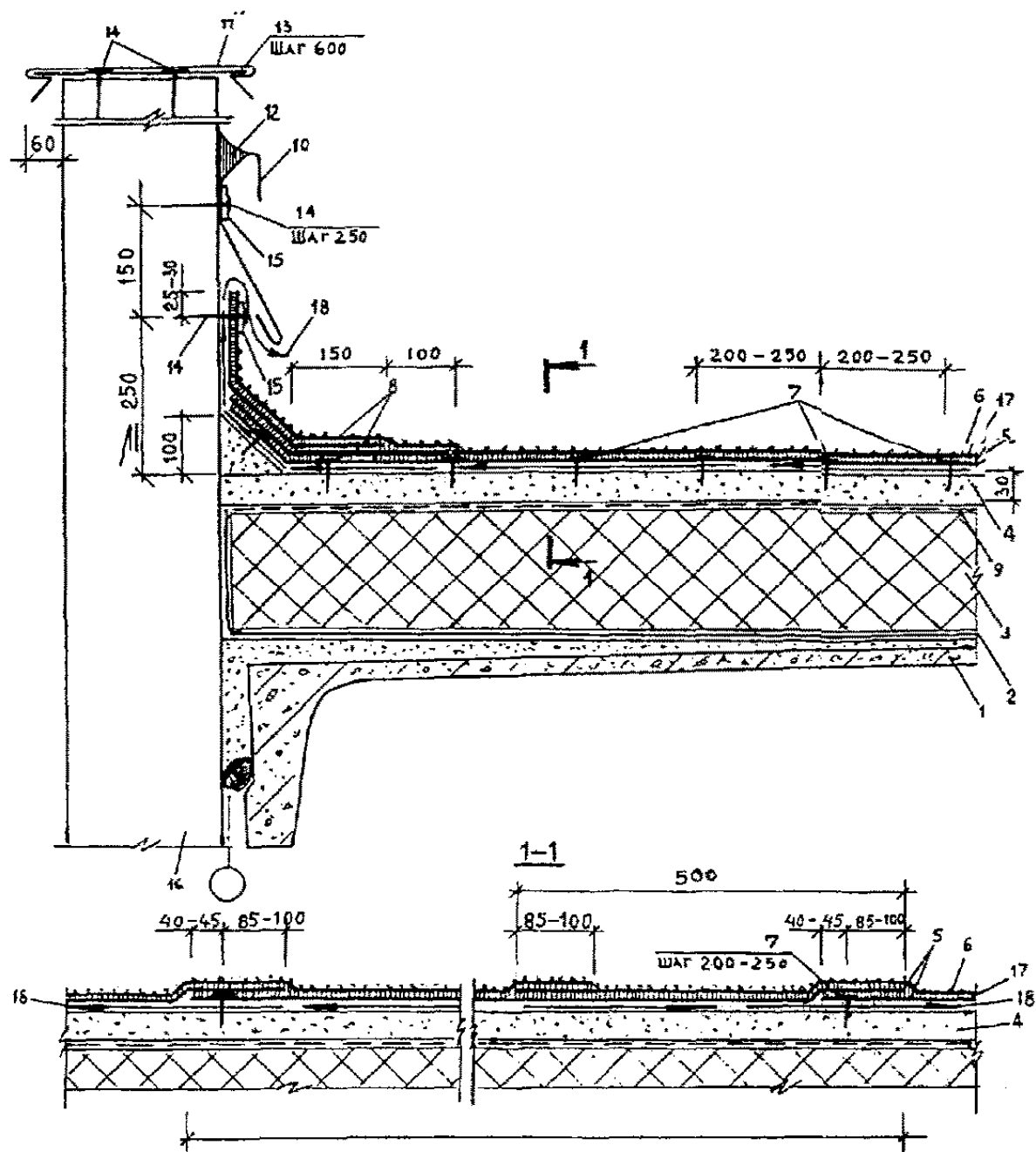
Рис. 2 Примыкание кровли к парапету (стене) при механическом закреплении нижнего слоя водоизоляционного ковра
