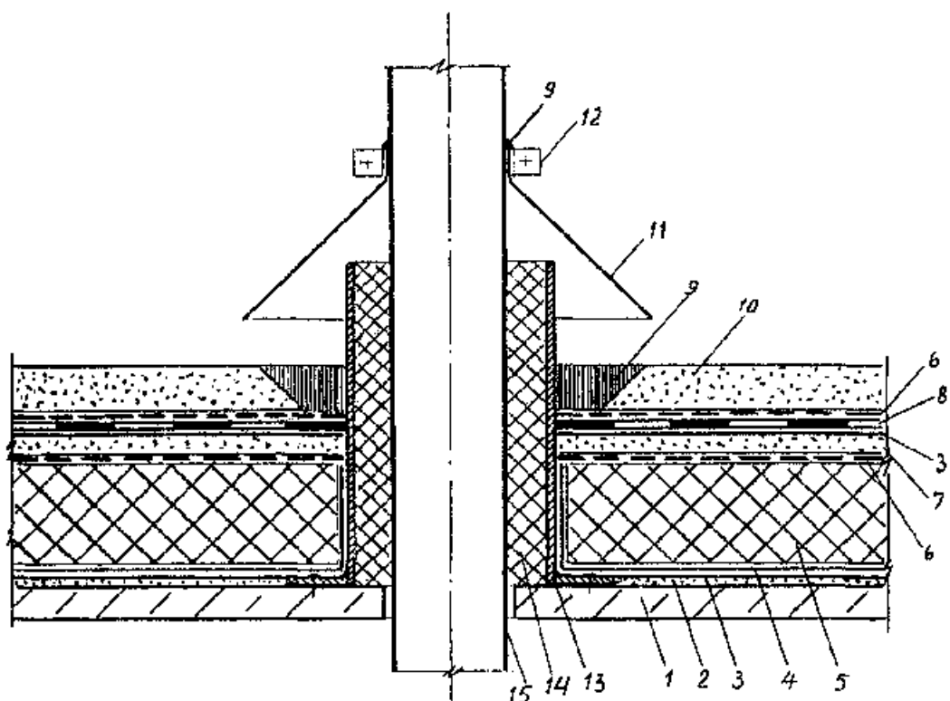
Рис. 3 Пропуск трубы через традиционную эксплуатируемую кровлю.
