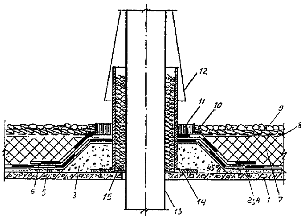
Рис. 4 Пропуск трубы через инверсионную эксплуатируемую кровлю.
