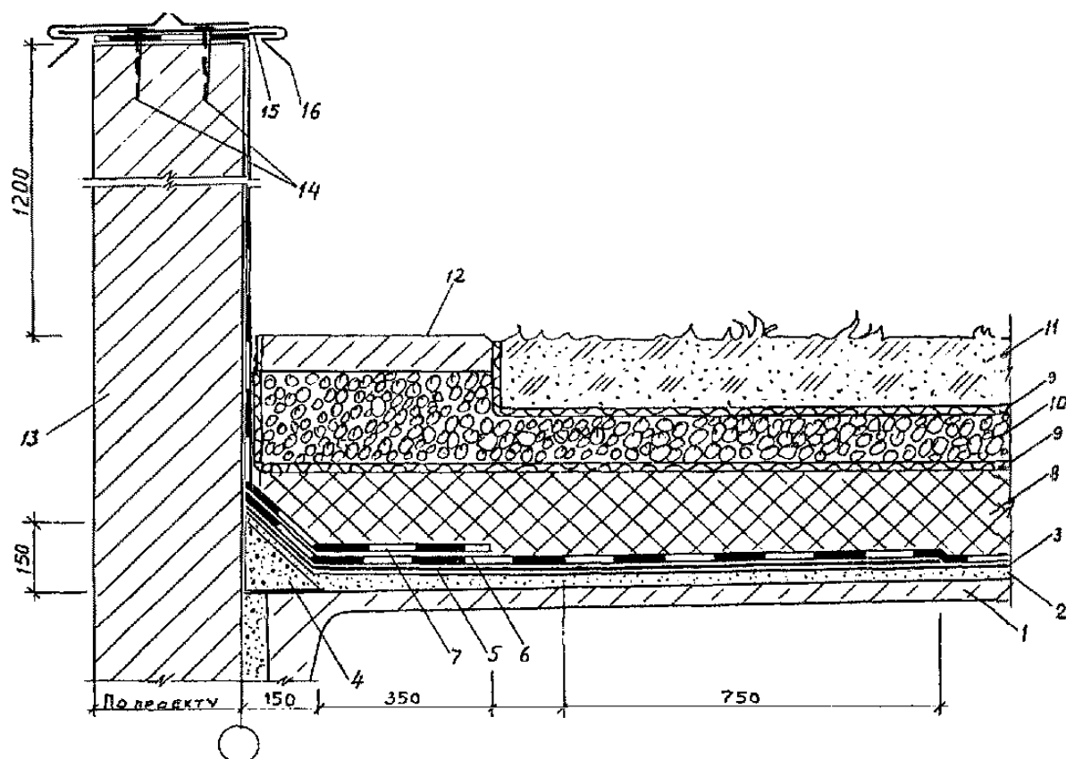
Рис. 9 Парапет стены при инверсионной эксплуатируемой кровле.
