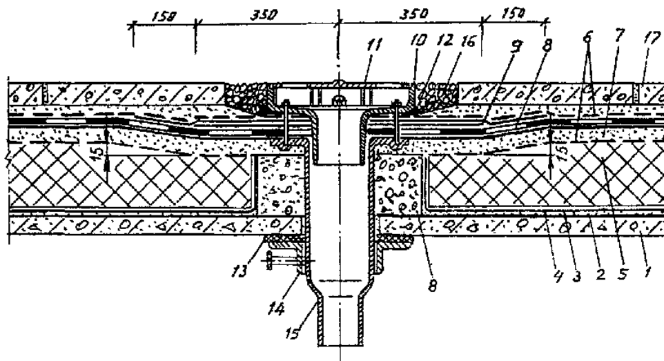
Рис. 10 Воронка внутреннего водостока при традиционной эксплуатируемой кровле.
