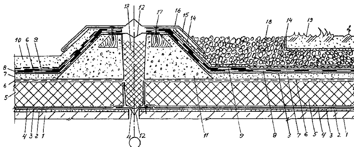
Рис. 5 Деформационный шов при традиционной эксплуатируемой кровле.
