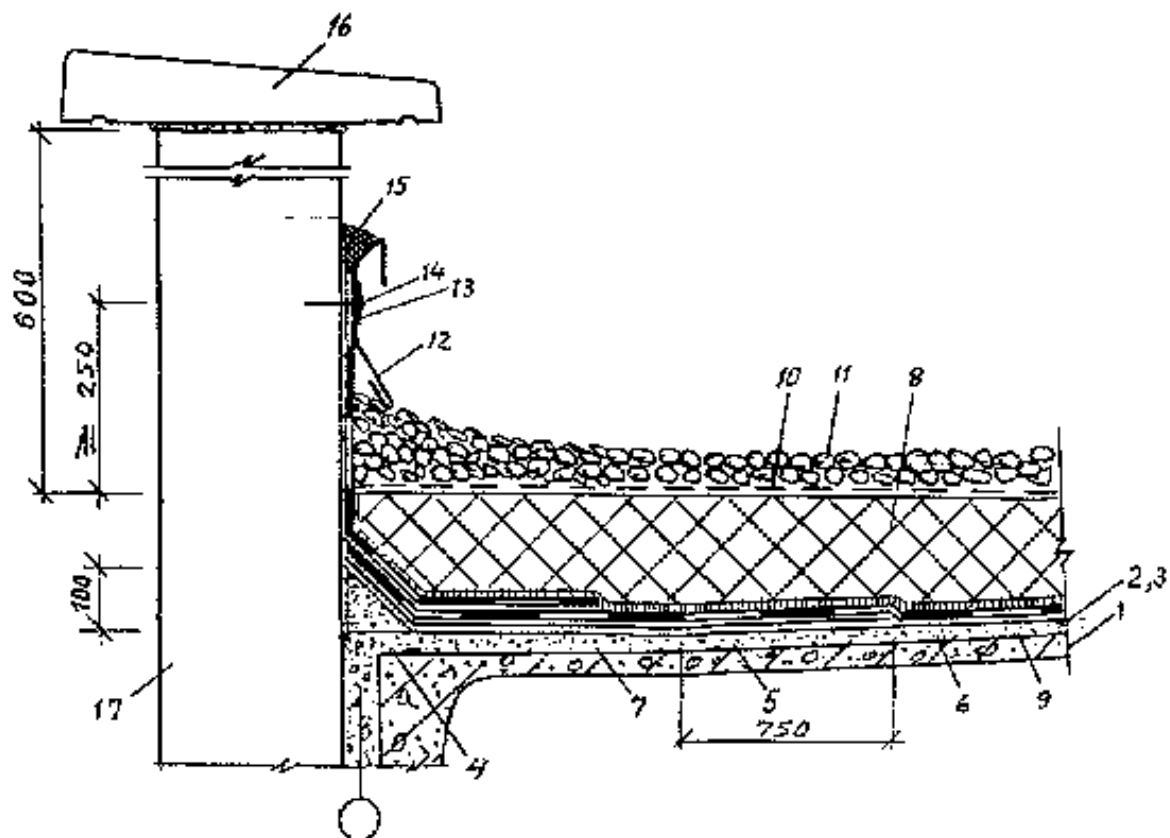
Рис. 8 Парапет продольной стены при инверсионной эксплуатируемой кровле
