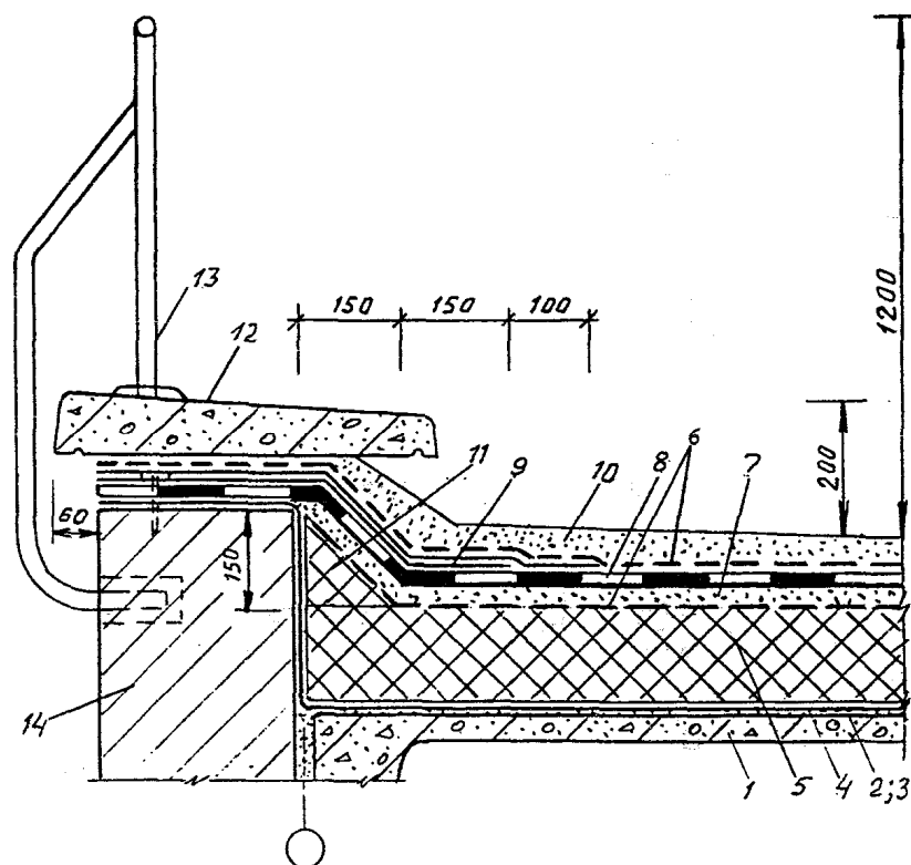
Рис. 7 Парапет продольной стены при традиционной эксплуатируемой кровле
