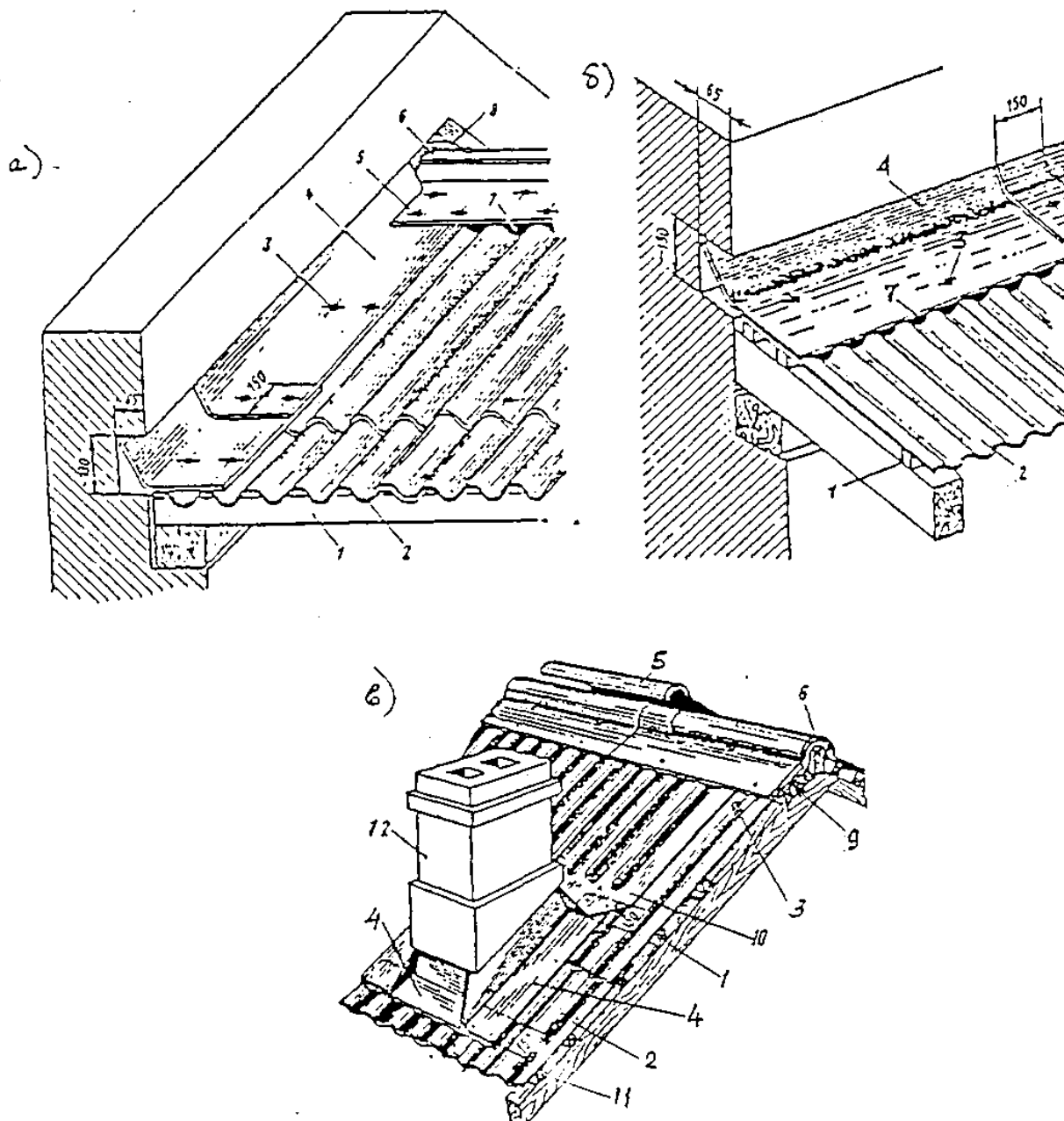
Рис. 21 Конструкция примыкания кровли из асбестоцементных волнистых листов к продольной (а) и поперечной (б) стенам и устройство воротника дымовой трубы (в)
