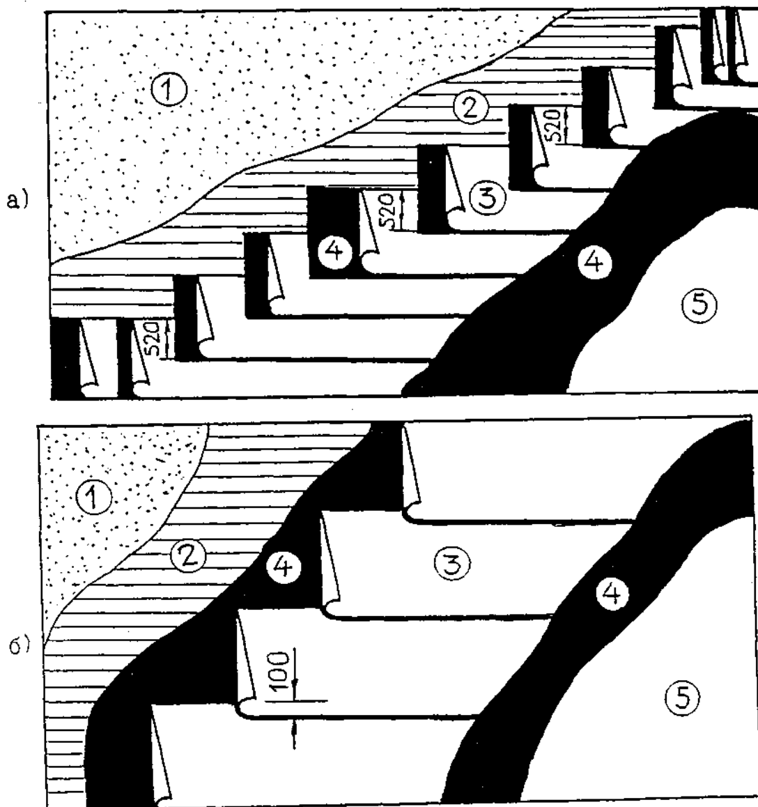
Рис. 17. Схема расположения слоев мастичного кровельного ковра а) с двумя армирующими слоями (ступенчатое расположение слоев); б) с одним армирующим слоем; 1 – основание под кровлю; 2 – грунтовка; 3 – армирующие слои; 4 – слои мастики; 5 – защитный (окрасочный) слой.
