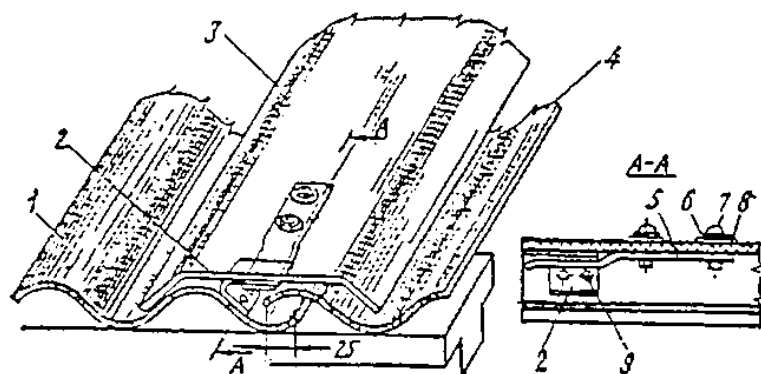
Рис. 22. Компенсационный шов
