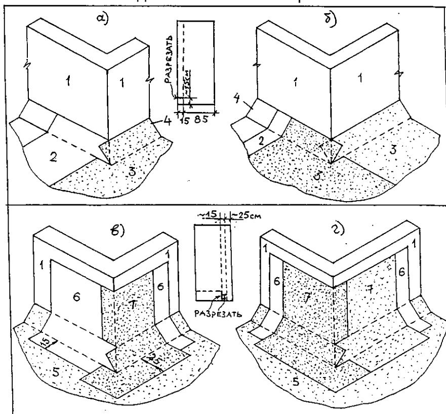
Рис. 13. Раскладка и раскрой полотнищ наплавляемого рулонного материала при устройстве кровельного ковра (а и б – основного, в и г – дополнительного) на поверхности внешнего угла, например, вентшахты
