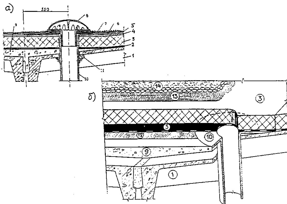
Рис. 5. Воронка внутреннего водостока
