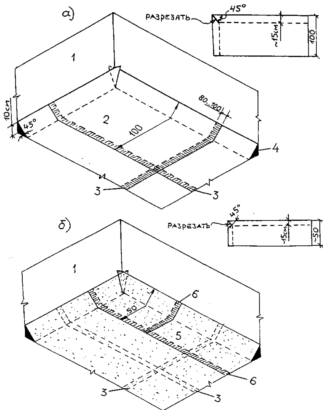
Рис.11 Раскладка и раскрой полотнищ наплавляемого рулонного материала (а - нижнего слоя; б - верхнего слоя) при устройстве основного кровельного ковра в углу парапета
