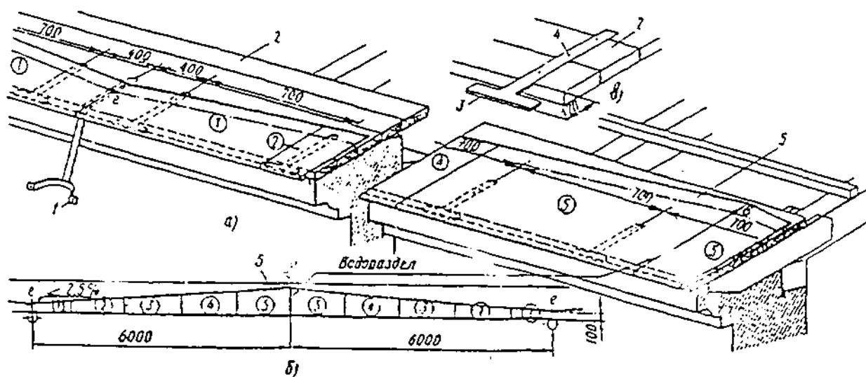
Рис. 28. Покрытие карнизного свеса
