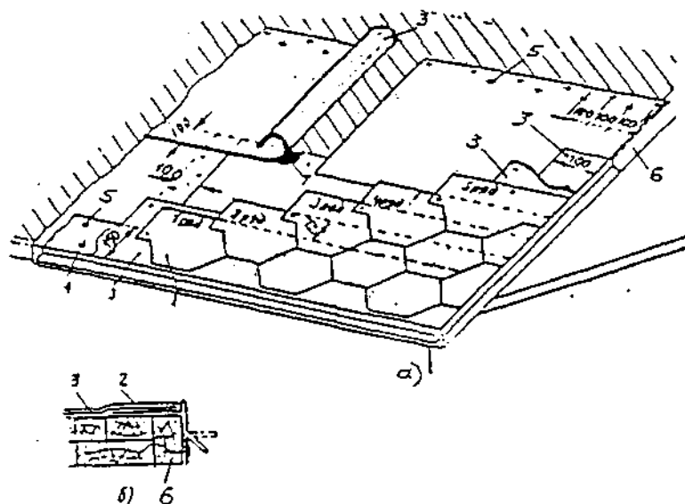
Рис. 25. Конструктивное решение кровли из битумных плиток (шинглс)
