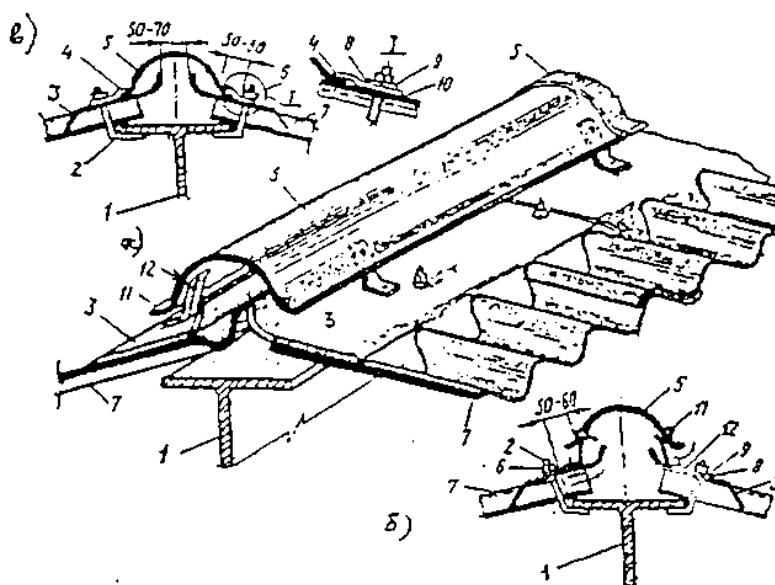
Рис. 23. Устройство коньков
