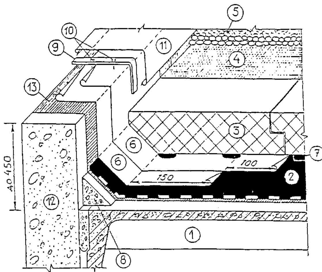
Рис. 1. Инверсионная кровля с теплоизоляцией из экструзионного пенопласта
