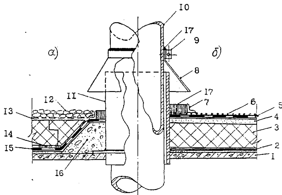
Рис. 4. Примыкание кровли к трубе
