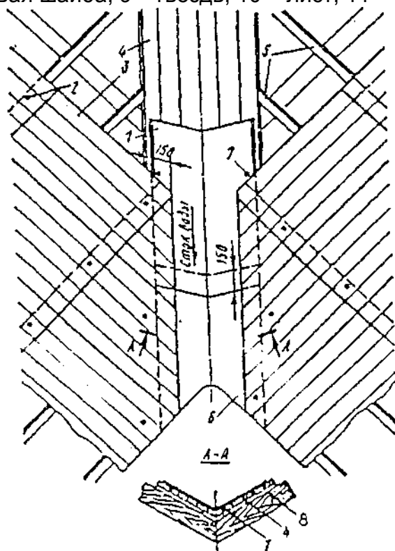
Рис.20. Устройство ендовы (разжелобка)
