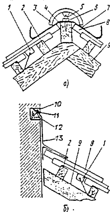
Рис. 26. Узлы черепичной кровли
