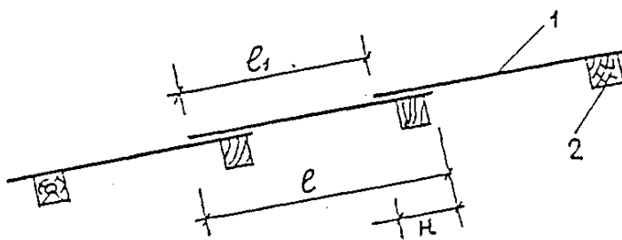
Рис. 5. 1 – асбестоцементный лист, металлический профнастил или металлочерепица; 2 – обрешетка.
