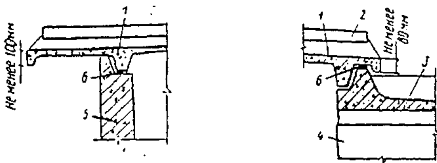
Рис. 37. Сливные свесы кровельной панели
