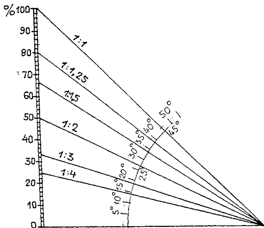
Рис. 3. График для определения величины уклона в %.
