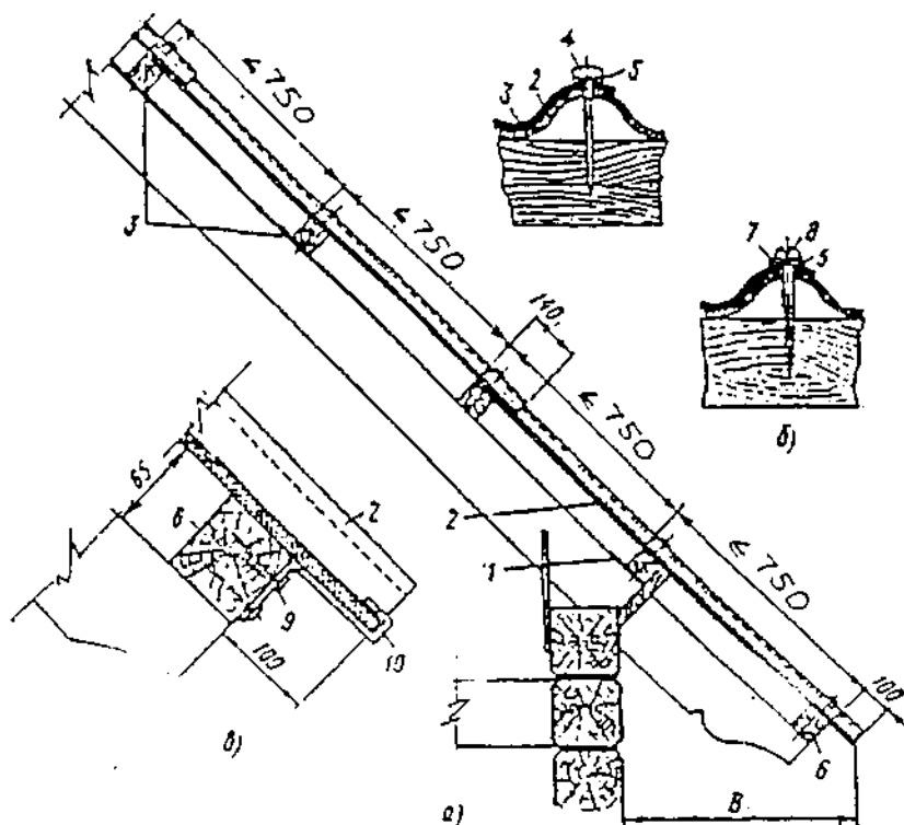
Рис. 18- Конструкция рядовой обрешетки и крепление асбестоцементных волнистых листов
