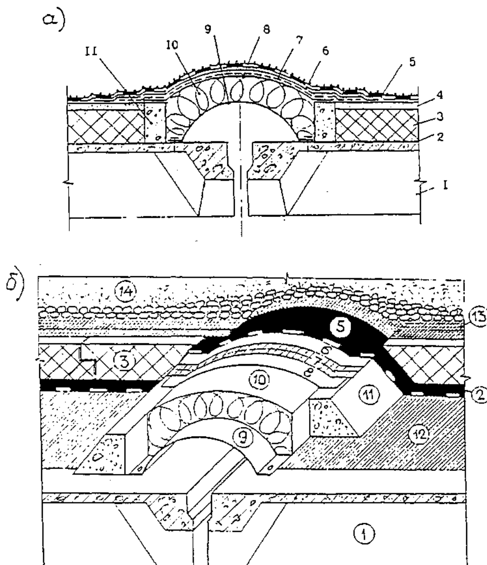
Рис. 6. Деформационный шов в покрытии
