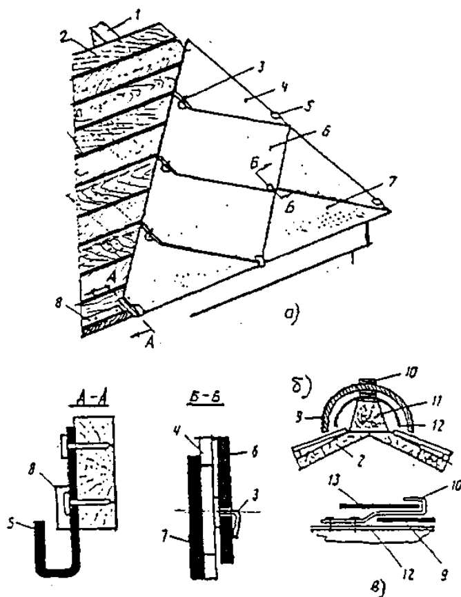
Рис. 24. Конструкция кровли из асбестоцементных плоских плиток
