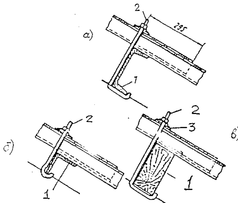
Рис 19.1 Способы крепления асбестоцементных волнистых листов к прогонам
