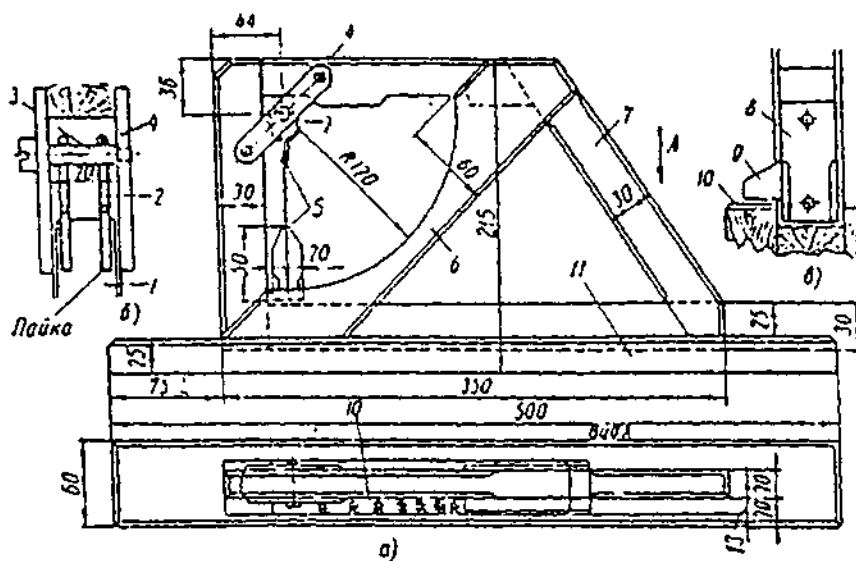
Рис. 2. а) боковой вид. б) – разрез шарнира, в) нижняя часть маятника. 1 – стальная пластина; 2 – проволочное кольцо; 3 – латунная ось; 4 – планка; 5 – маятник; 6 – направляющая; 7 – рамка; 8 – груз; 9 – указатель; 10 – шкала; 11 – опорная рейка.
