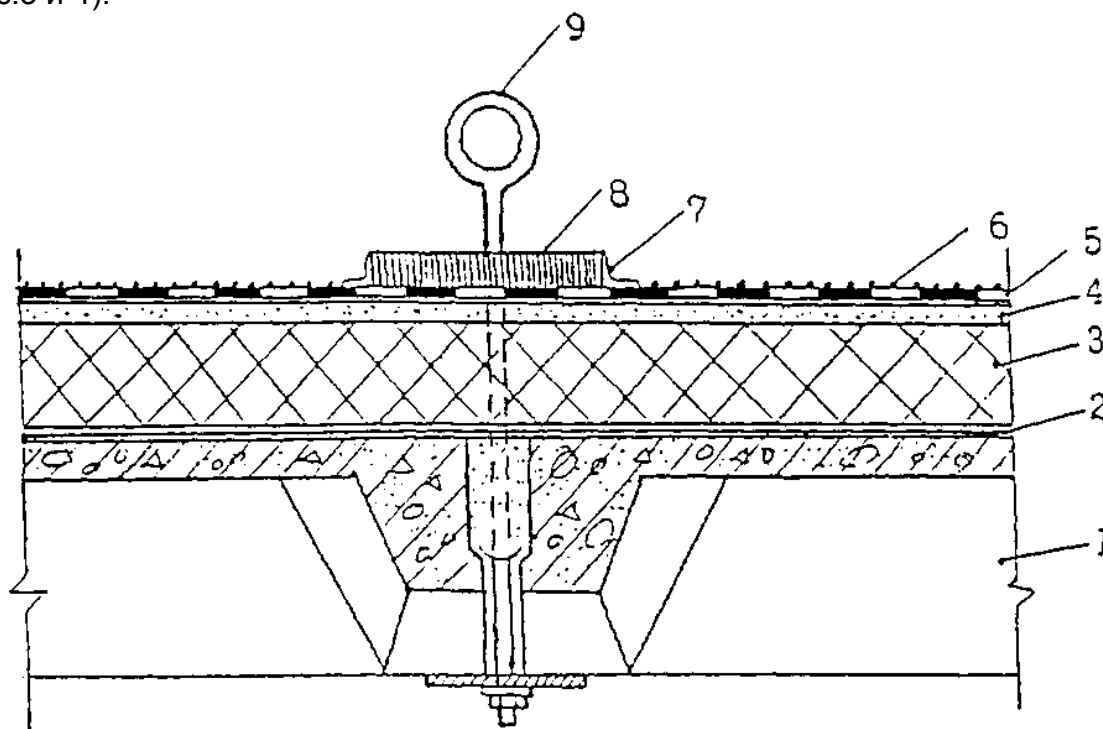
Рис. 3. Пропуск анкера через водоизоляционный ковёр
