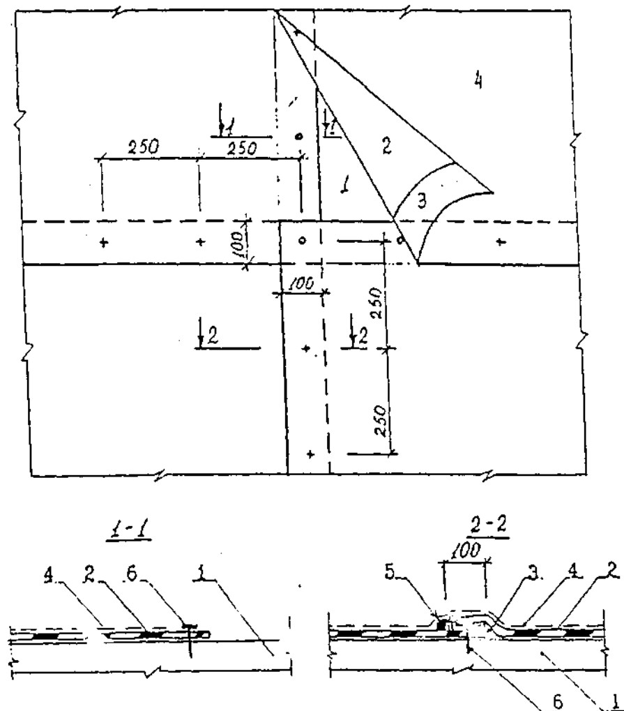
Рис. 16. Выполнение шва внахлестку
