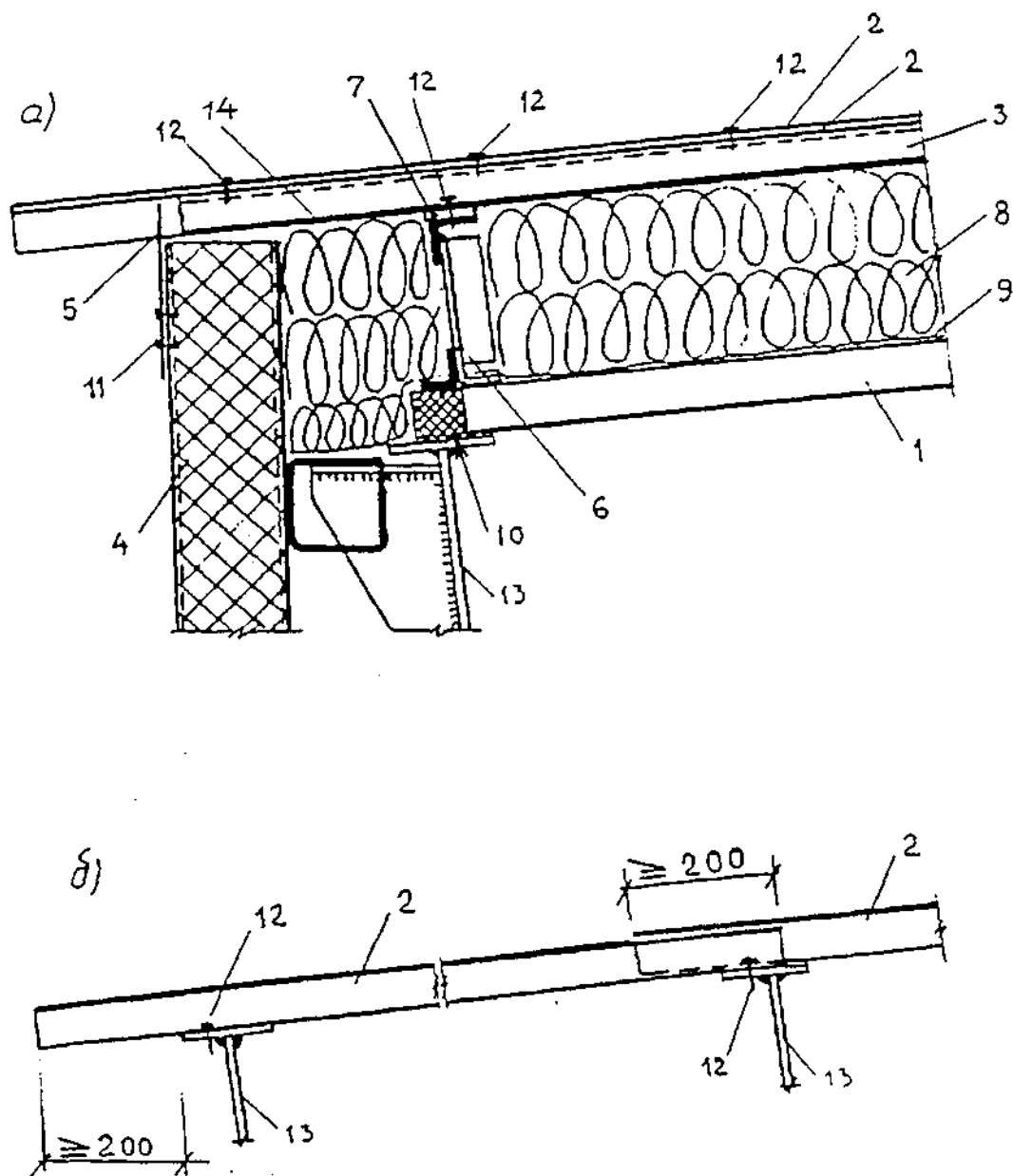
Рис. 31 Карниз кровли из металлического профнастила
