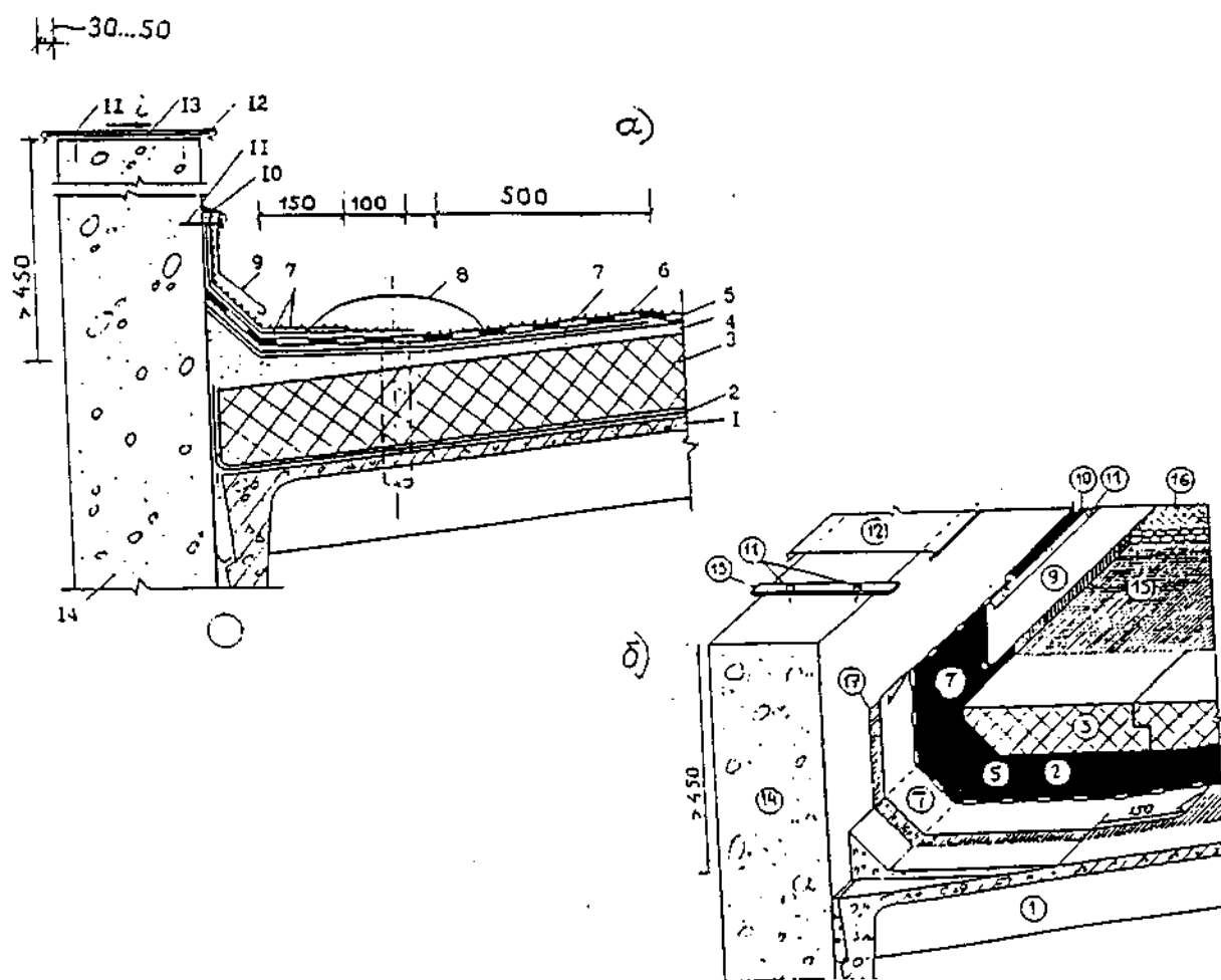
Рис. 8. Примыкание кровли к парапету высотой более 450 мм
