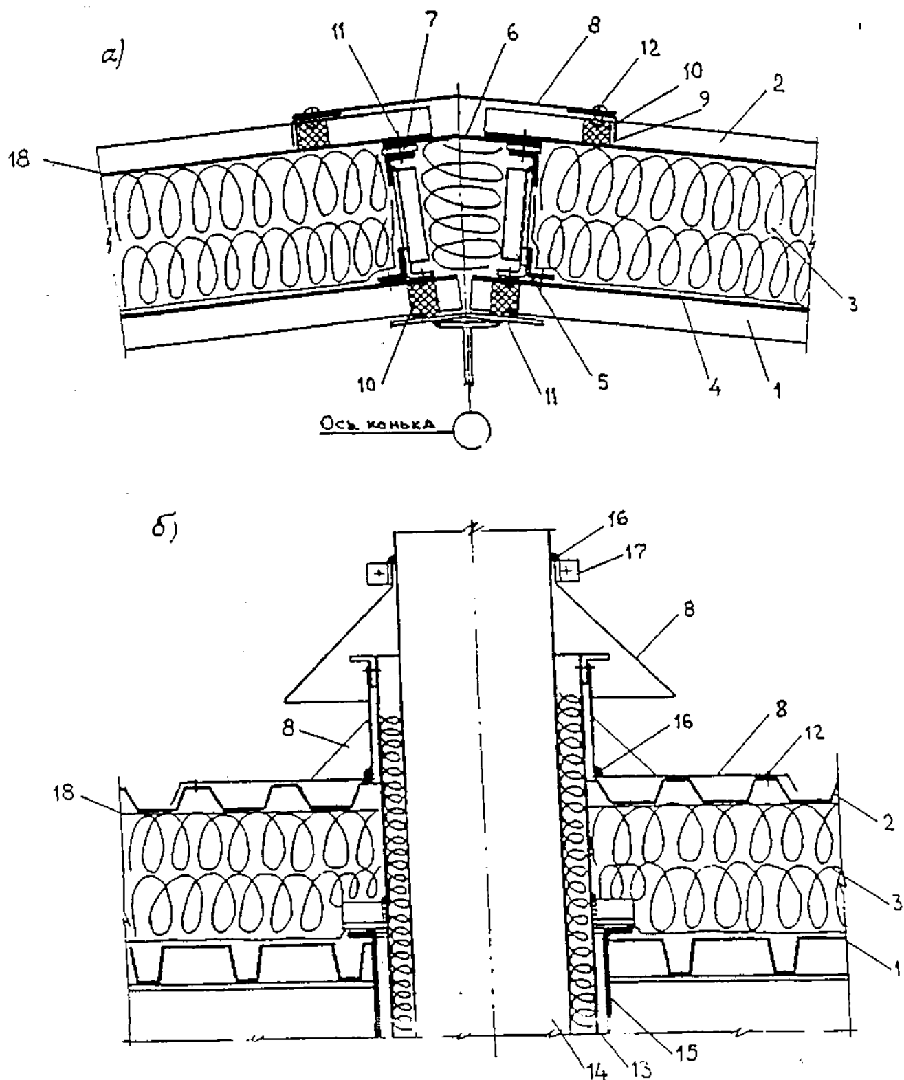
Рис 32 Кровля из металлического профнастила
