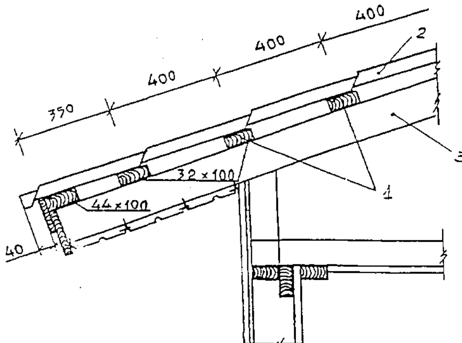
Рис. 34. Конструкция обрешетки под кровлю из металлочерепицы
