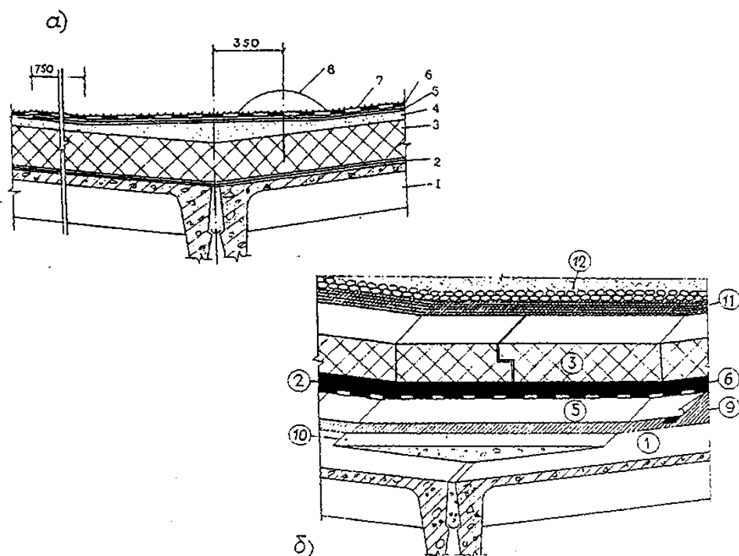
Рис. 10. Ендова кровли
