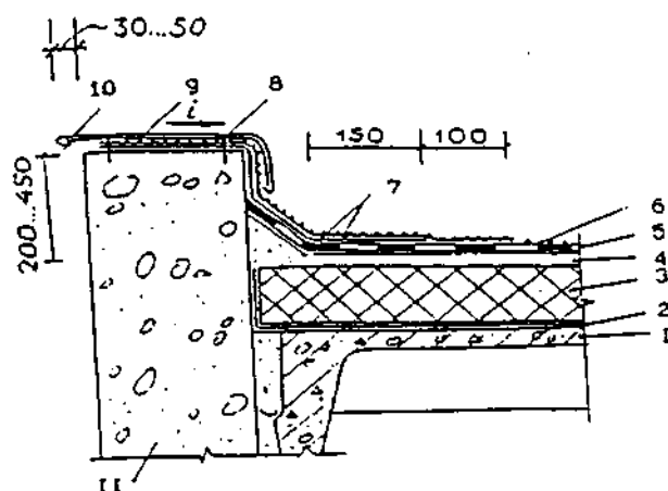
Рис. 7. Примыкание кровли к парапету высотой до 450 мм
