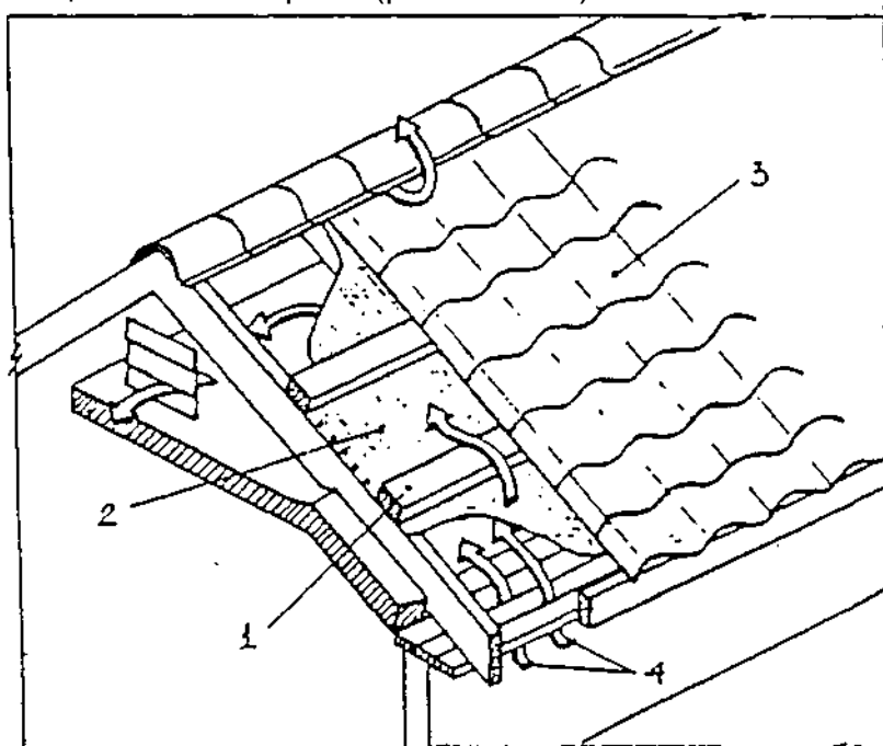
Рис. 33. Конструкция крыши с кровлей из металлочерепицы
