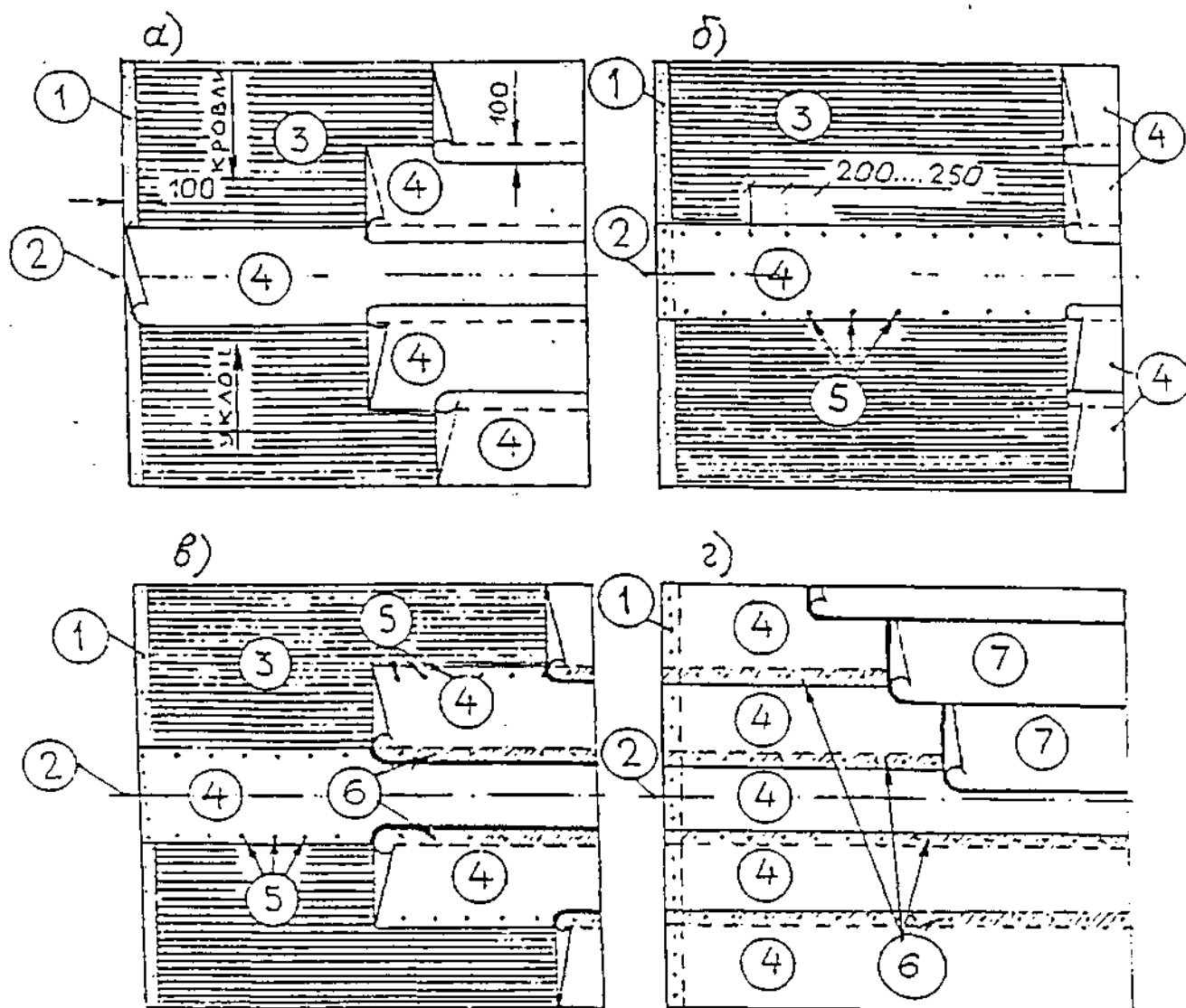
Рис.14. Последовательность (а, б, в, г) раскладки рулонных материалов при устройстве водоизоляционного ковра с механическим закреплением нижнего слоя 1 – переходной наклонный бортик; 2 – линия водораздела; 3 – основание под кровлю; 4 – нижний слой водоизоляционного ковра; 5 – шайбы с дюбелями; 6 – наклейка полотнищ в местах нахлесток; 7 – верхний (второй) слой водоизоляционного ковра
