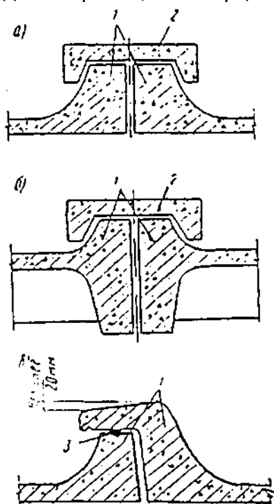
Рис. 36. Конструкции стыков кровельных панелей
