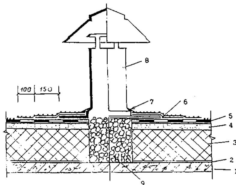
Рис. 2. Вентиляционный патрубок
