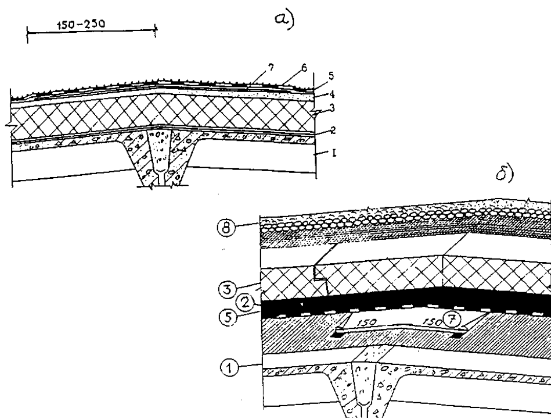
Рис. 9. Конек кровли
